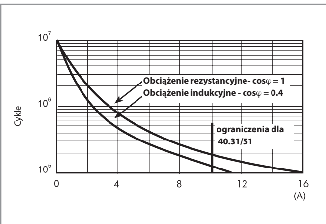
F 40.5 - Trwałość łączeniowa (dla AC) w funkcji prądu na zestykach Typ 40.11 (strona 5)
