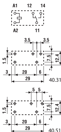
Rysunek otworów montażowych Długość pinów 5.3 mm dla gniazd i obwodów drukowanych
