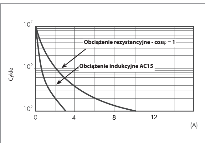
F 40.6 - Trwałość łączeniowa (dla AC) w funkcji prądu na zestykach Typ 40.62 (strona 5)
