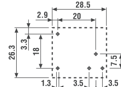
Rysunek otworów montażowych
