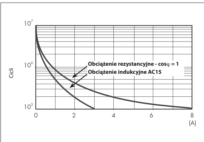
F 40.4 - Trwałość łączeniowa (dla AC) w funkcji prądu na zestykach Typ 40.52 (strona 4)
